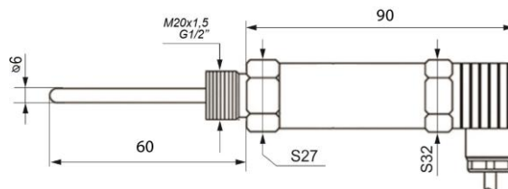
Рисунок 1 – Термопреобразователь с цифровым выходом T.Pt – RS–DIN – 6 – 60 – (-70/+200)
